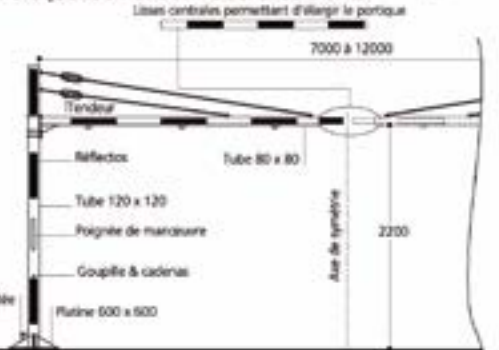
4 Portique pivotant
