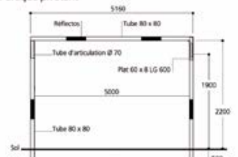
4 Portique pivotant
