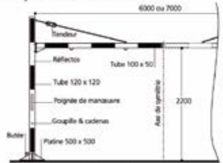
3 Portique tournant universel avec tirants
