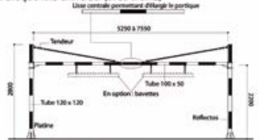
2 Portique fixe universel (sans tirants)
