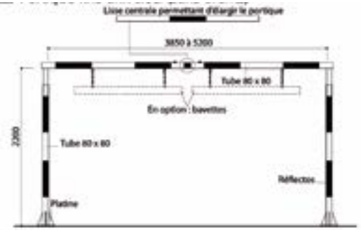
1 Portique fixe universel (avec tirants)
